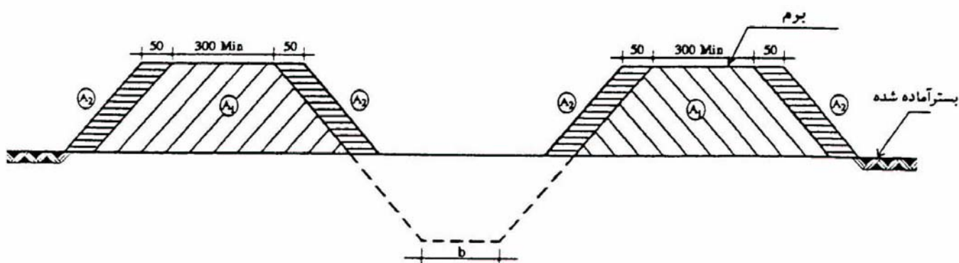
شکل ۴. شمای مقطع خاکریزی
